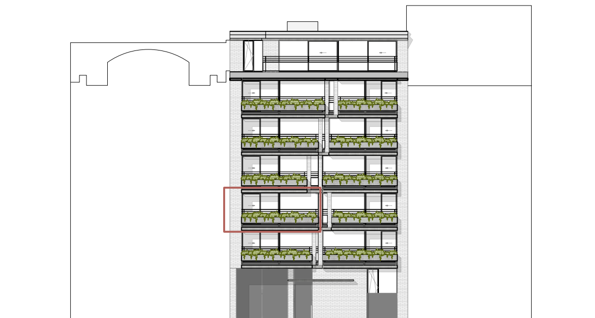
Voorgevel Floraliënlaan
